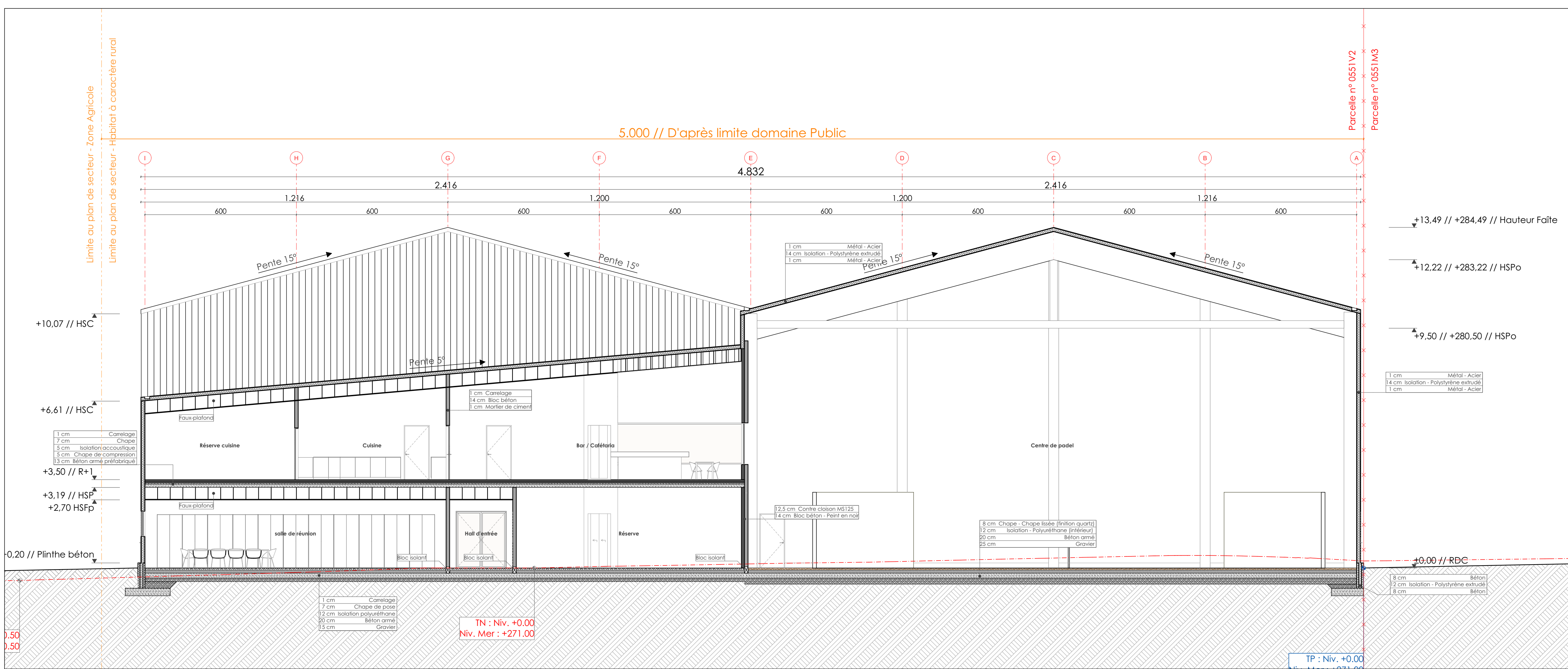
Coupe BB' Ech. 1:100
