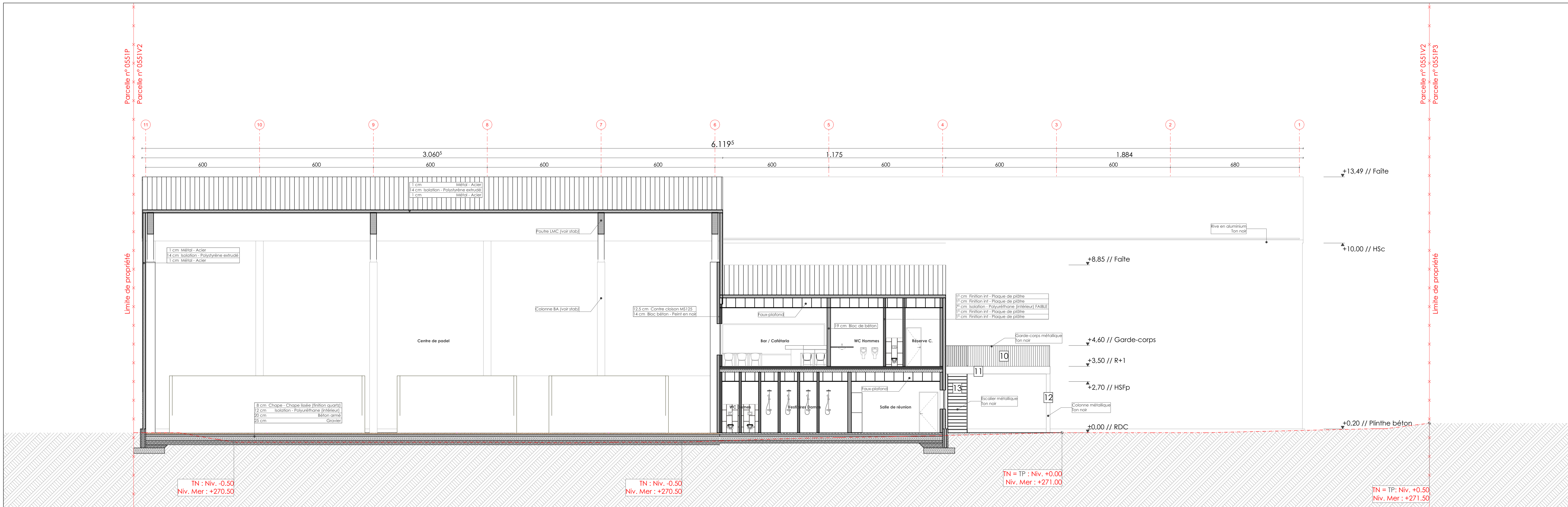
Coupe AA' Ech. 1:100
